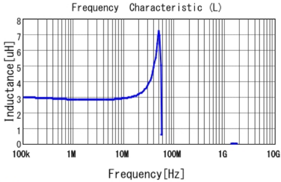
■ 1273AS-H-3R3N L
