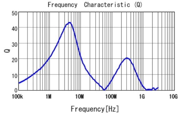
■ 1273AS-H-3R3N Q
