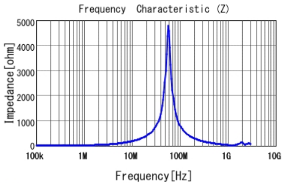
■ 1273AS-H-3R3N |Z|
